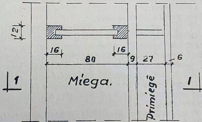
Plāns. MIEGU IRENGĪMAS. M 1:25 Paulauskiā A., Tauzu k.
